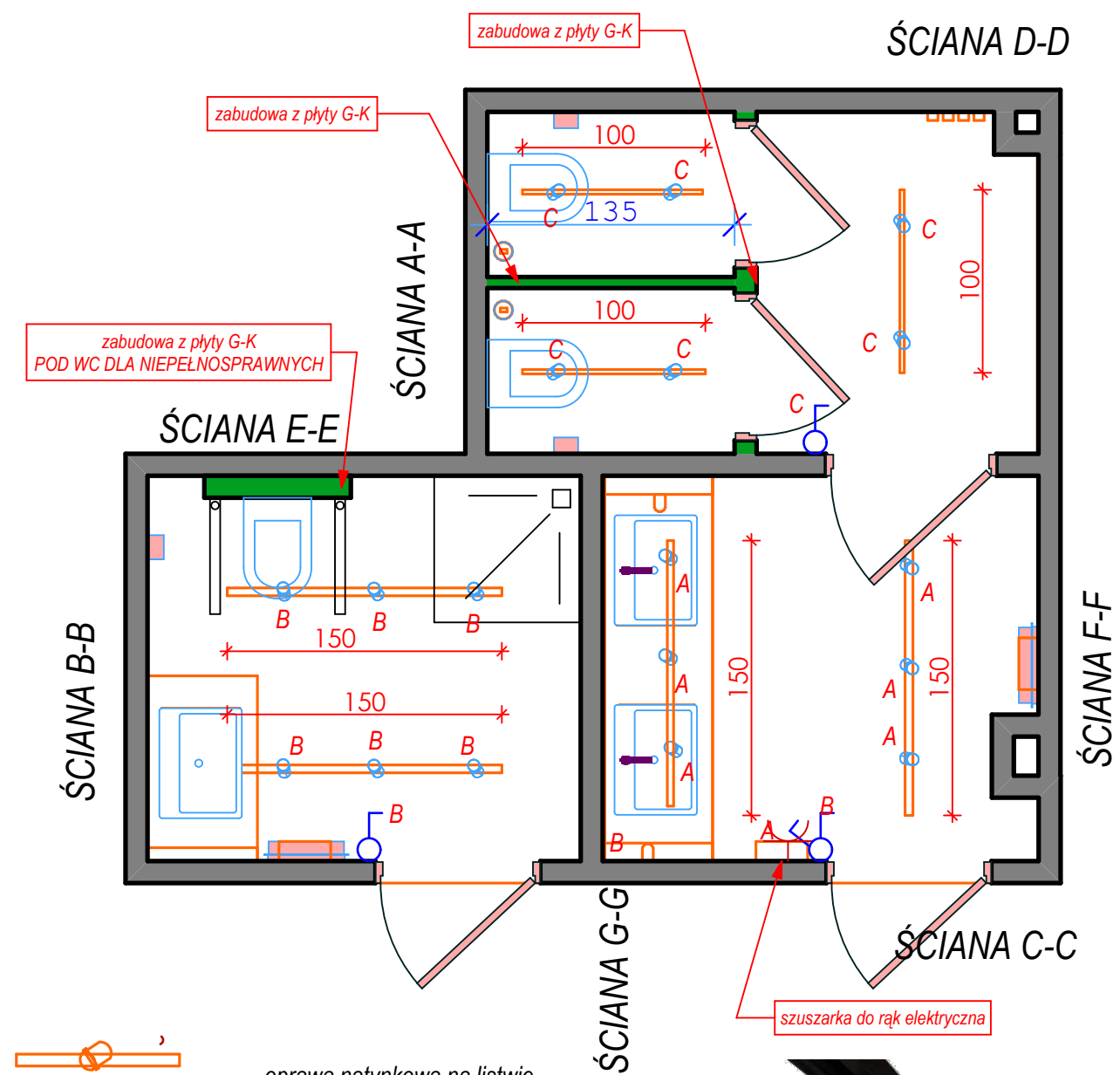
oprawa natynkowa kolor biały
