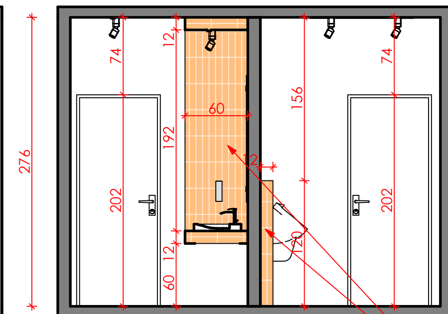
ŚCIANA E-E
