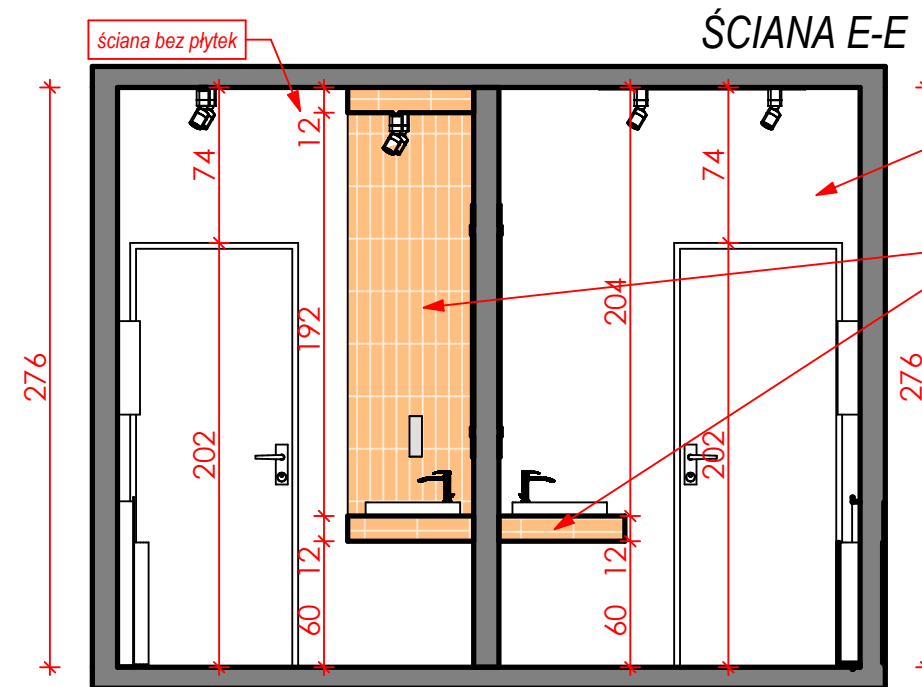
ŚCIANA E-E
