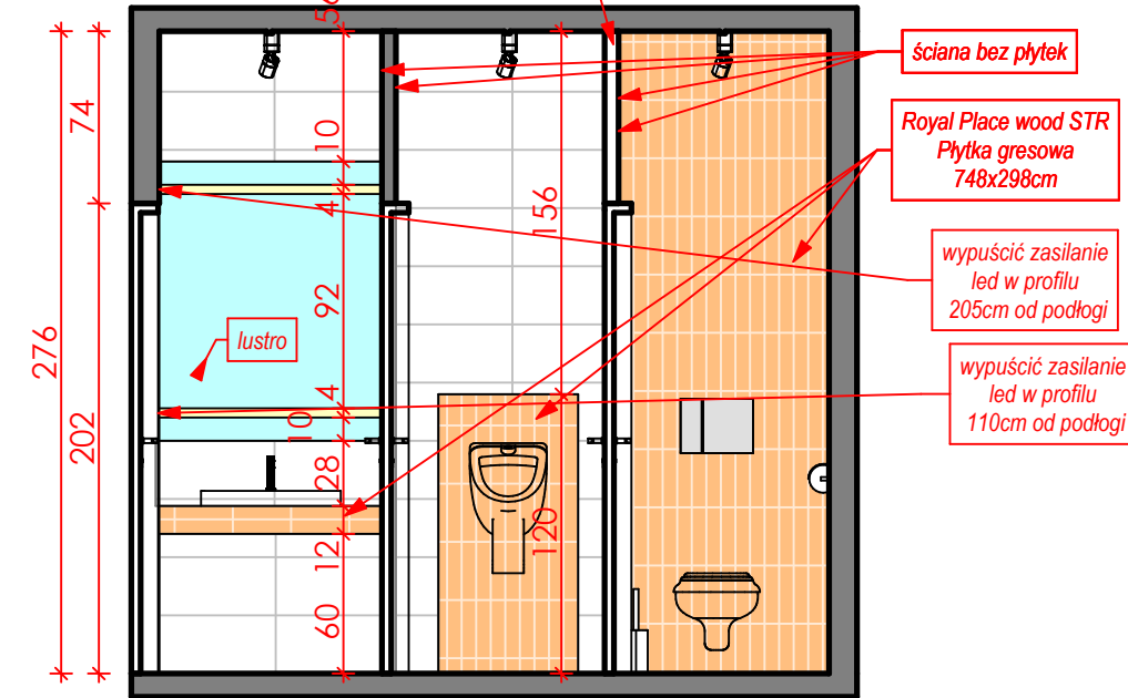
ŚCIANA F-F
