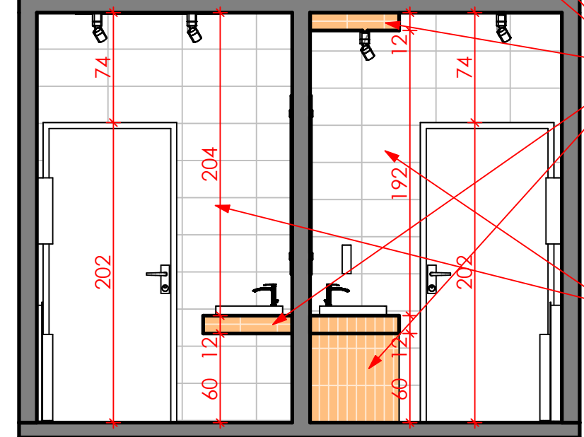
ŚCIANA C-C
