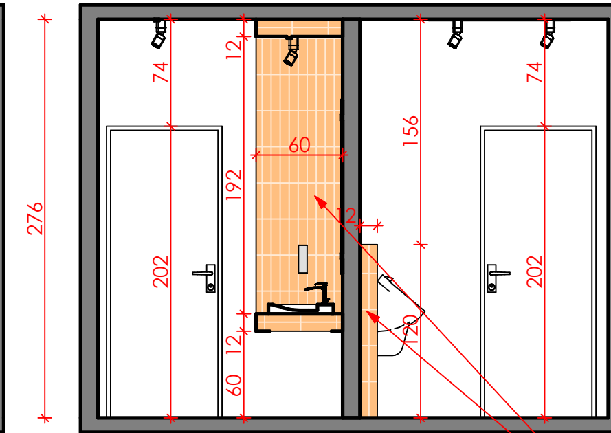
ŚCIANA E-E
