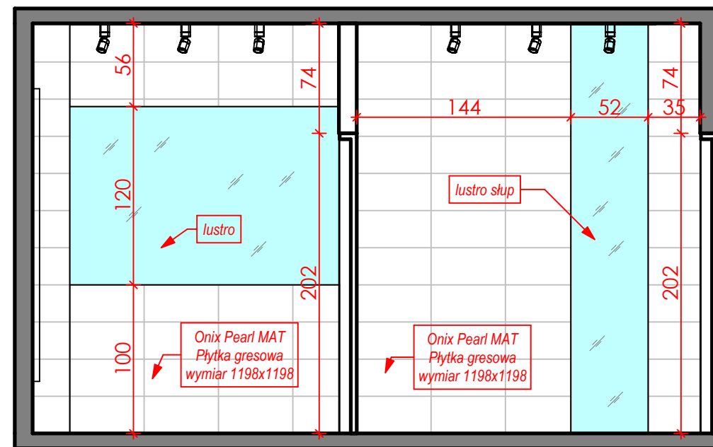
ŚCIANA E-E
