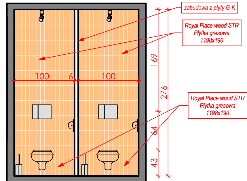
ŚCIANA B-B
