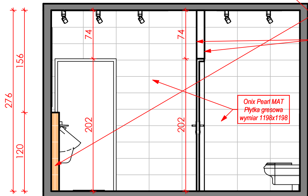
ŚCIANA I-I
