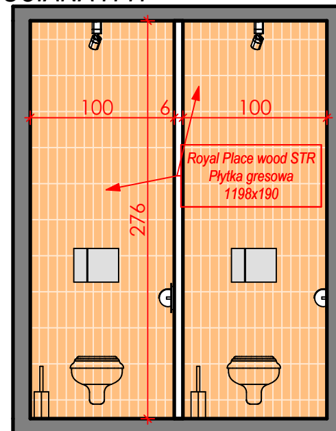
ŚCIANA H-H
