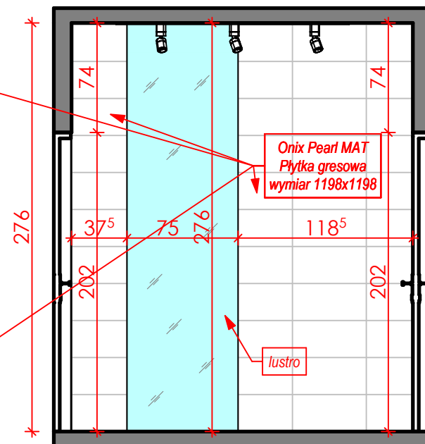
ŚCIANA H-H
