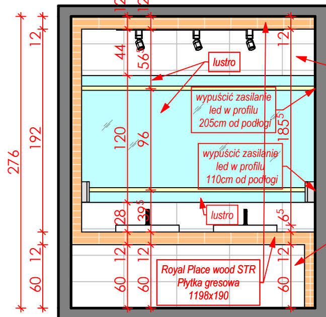
ŚCIANA E-E
