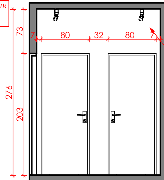
ŚCIANA F-F
