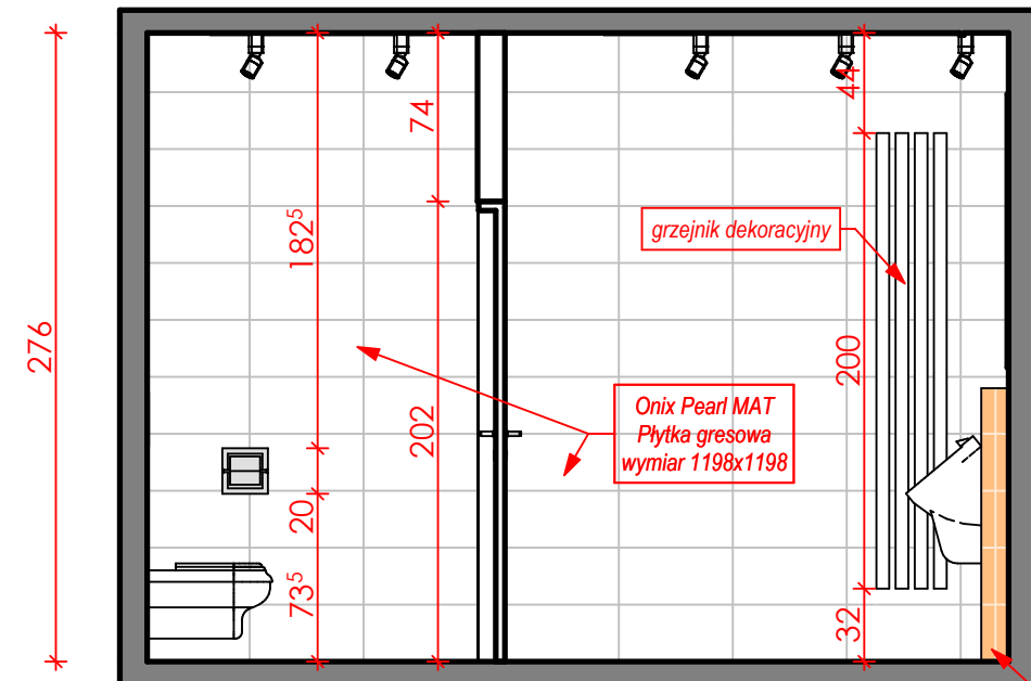
ŚCIANA E-E
