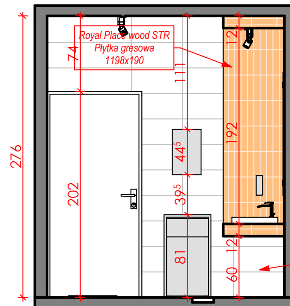
ŚCIANA G-G
