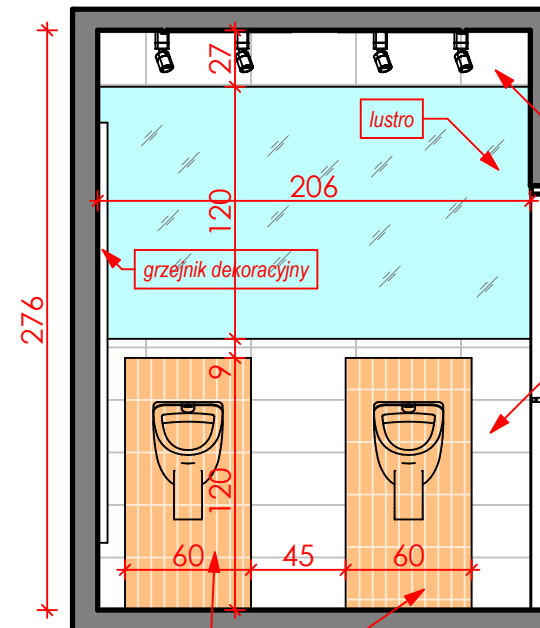
ŚCIANA G-G
